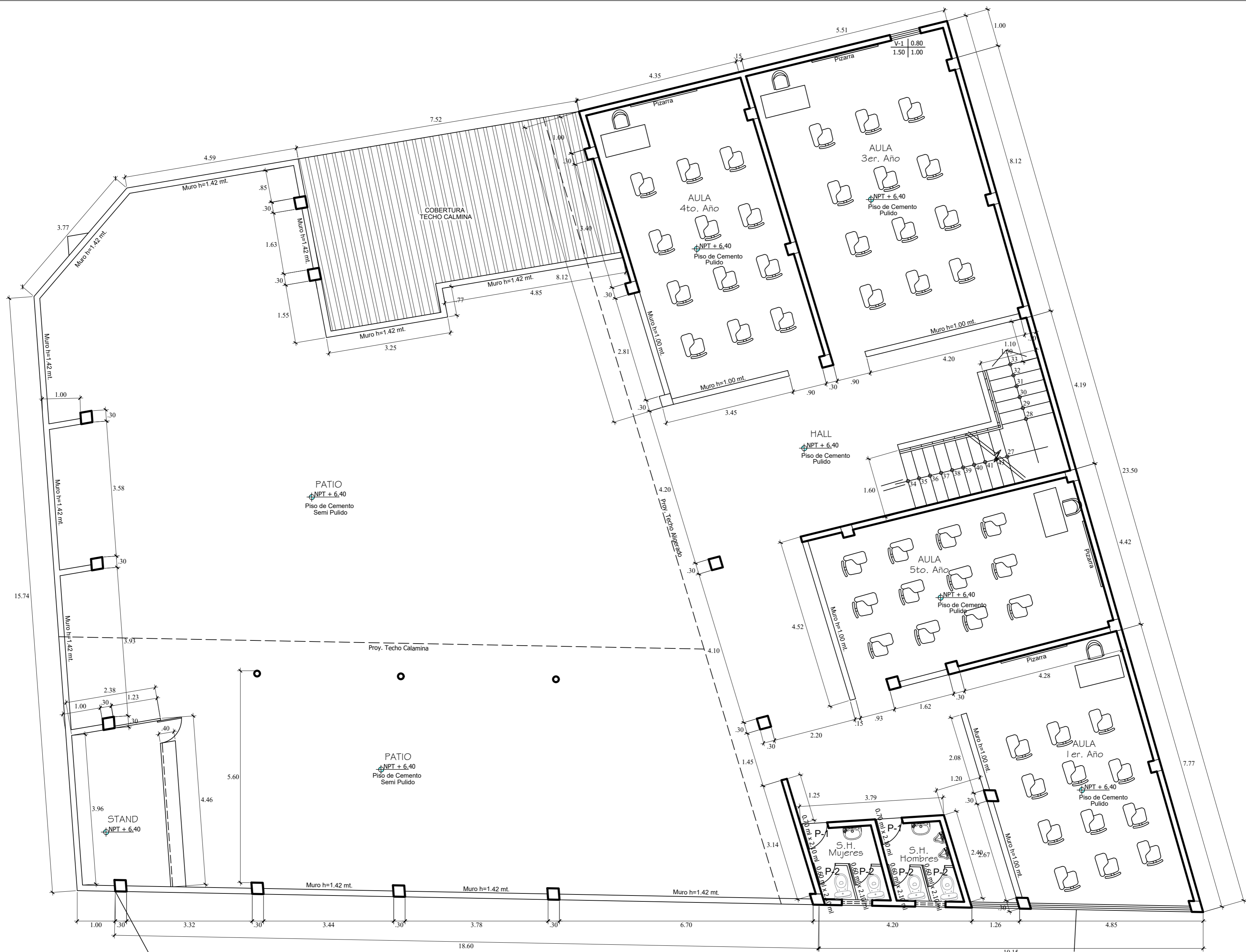
PLANTA 3° PISO ESC: 1/50
